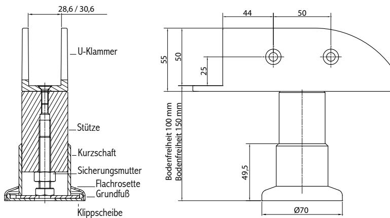
Darstellung MW2.4/28
